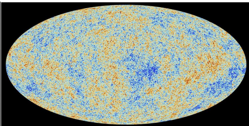
Fond diffus cosmologique (satellite Planck)
