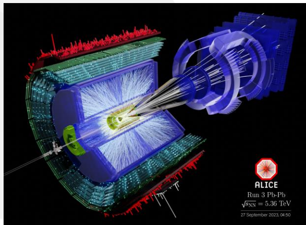
Collisions de particules au CERN Genève
