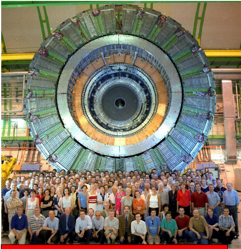
2001 : collaboration Delphi devant le détecteur
