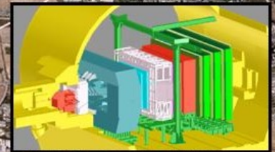
LHCb
