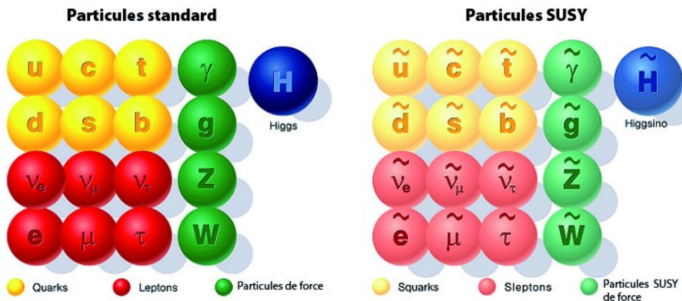
supersymétrie
