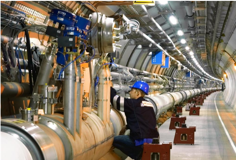
ligne cryogénique avant la pose des aimants
