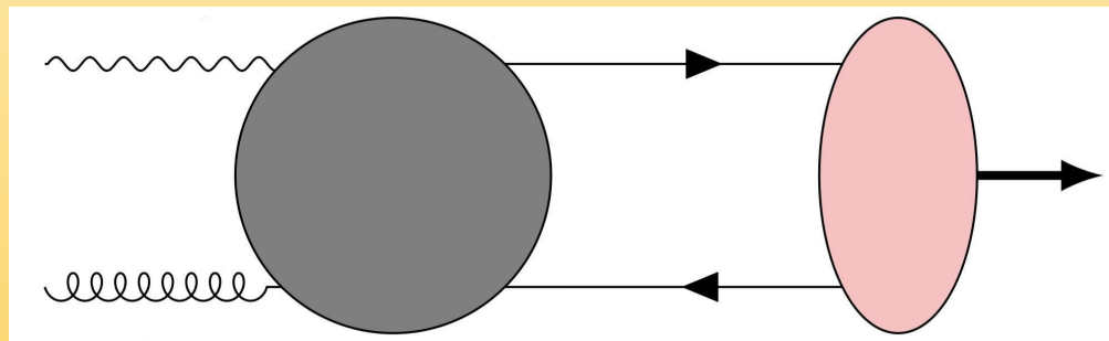
Quarkonium Production
