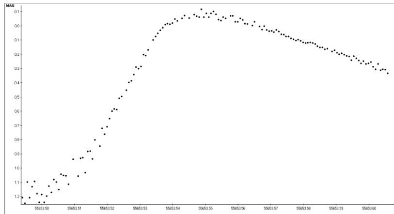
Courbe de variation photométrique obtenue après traitement des images et exploitation des données de RR Leo © S. Génard et al.
