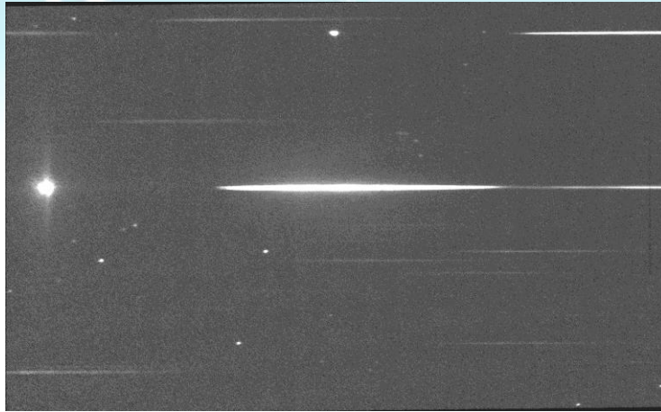
Etude de l'étoile Mu_Leo Lycée Jean Moulin Béziers, acd. Montpellier
