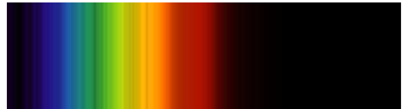
Etude de l'étoile Mu_Leo Lycée Jean Moulin Béziers, acd. Montpellier
