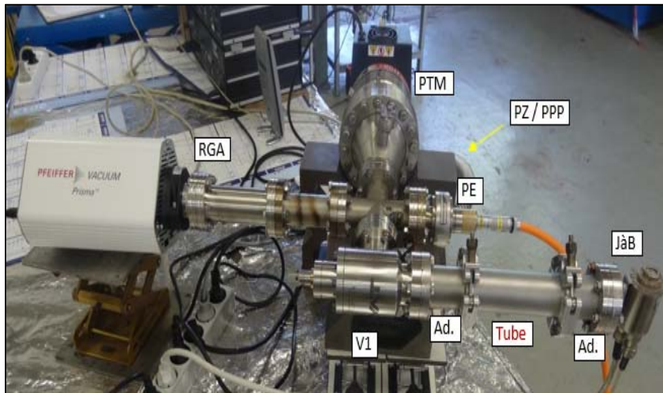
Montage de mesure du taux de dégazage
