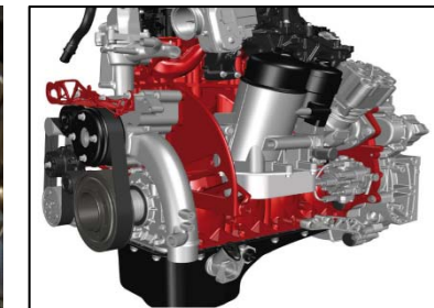
525 \rightarrow 120 kg - Moteur de Renault Trucks - 840 \rightarrow 640 pièces
