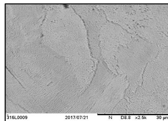
Microstructure en grains, taille \approx 50 \mu\text{m}
