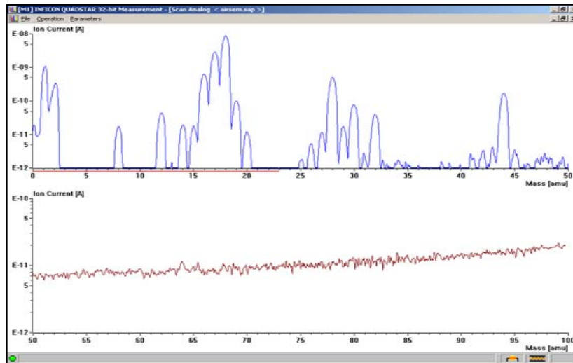
Spectres de masse
