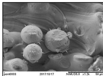
MEB - échelle 50 \mu\text{m}
