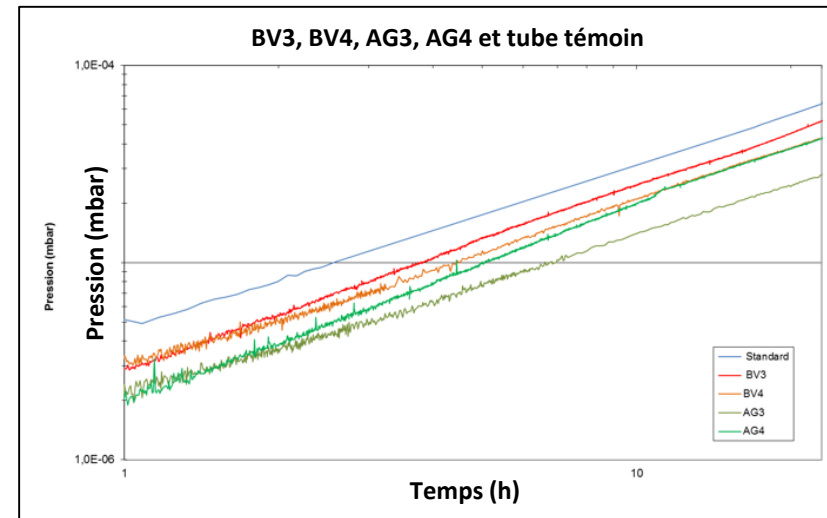
Courbes de remontée de pression
