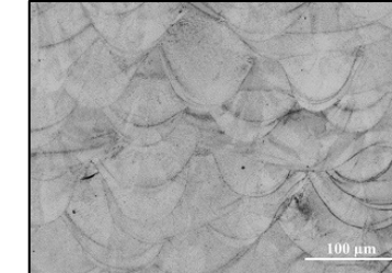
Microstructure en écailles, taille \approx 150 \mu\text{m}
