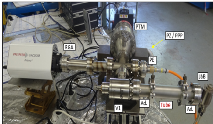
Montage de mesure du taux de dégazage
