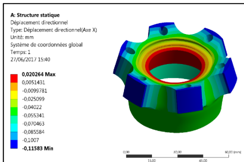
Calcul éléments finis ANSYS
