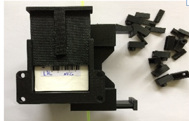
Dispositif de calibration SoLid 26 h de fabrication - 13 pièces - 58 €
