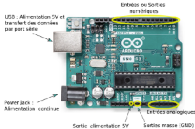
Microcontrôleur
