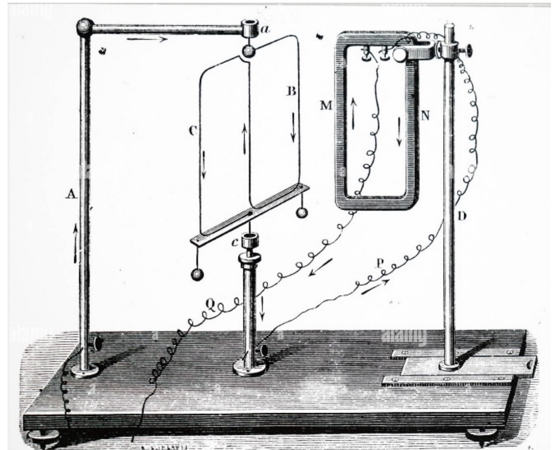
L'expérience d'Ampère
