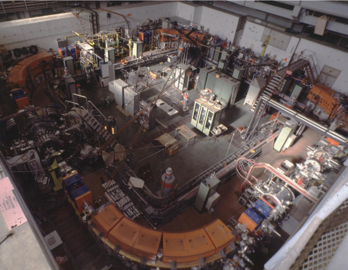
L'anneau LEAR d'antiprotons à basse énergie
